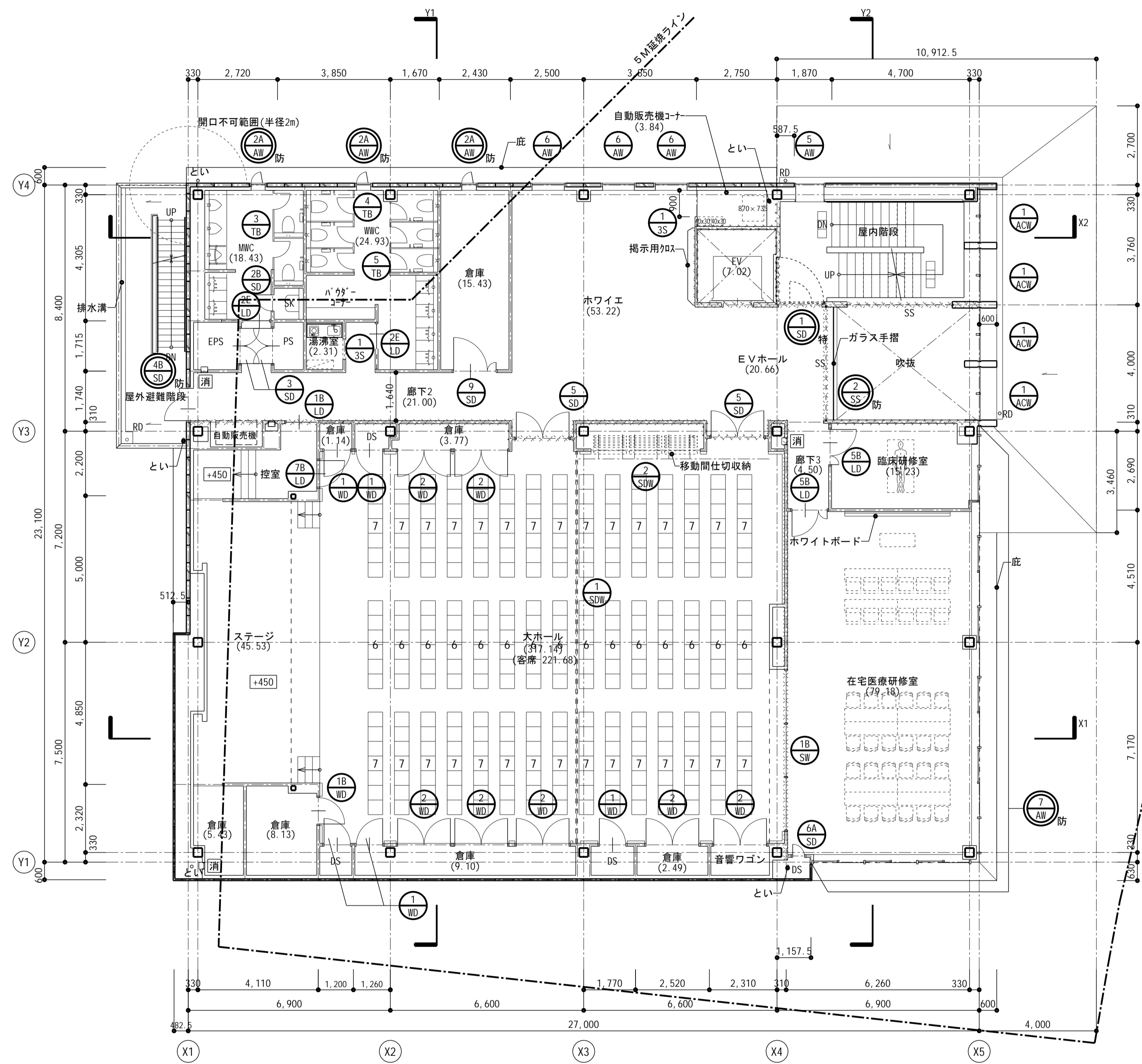
2階平面図
