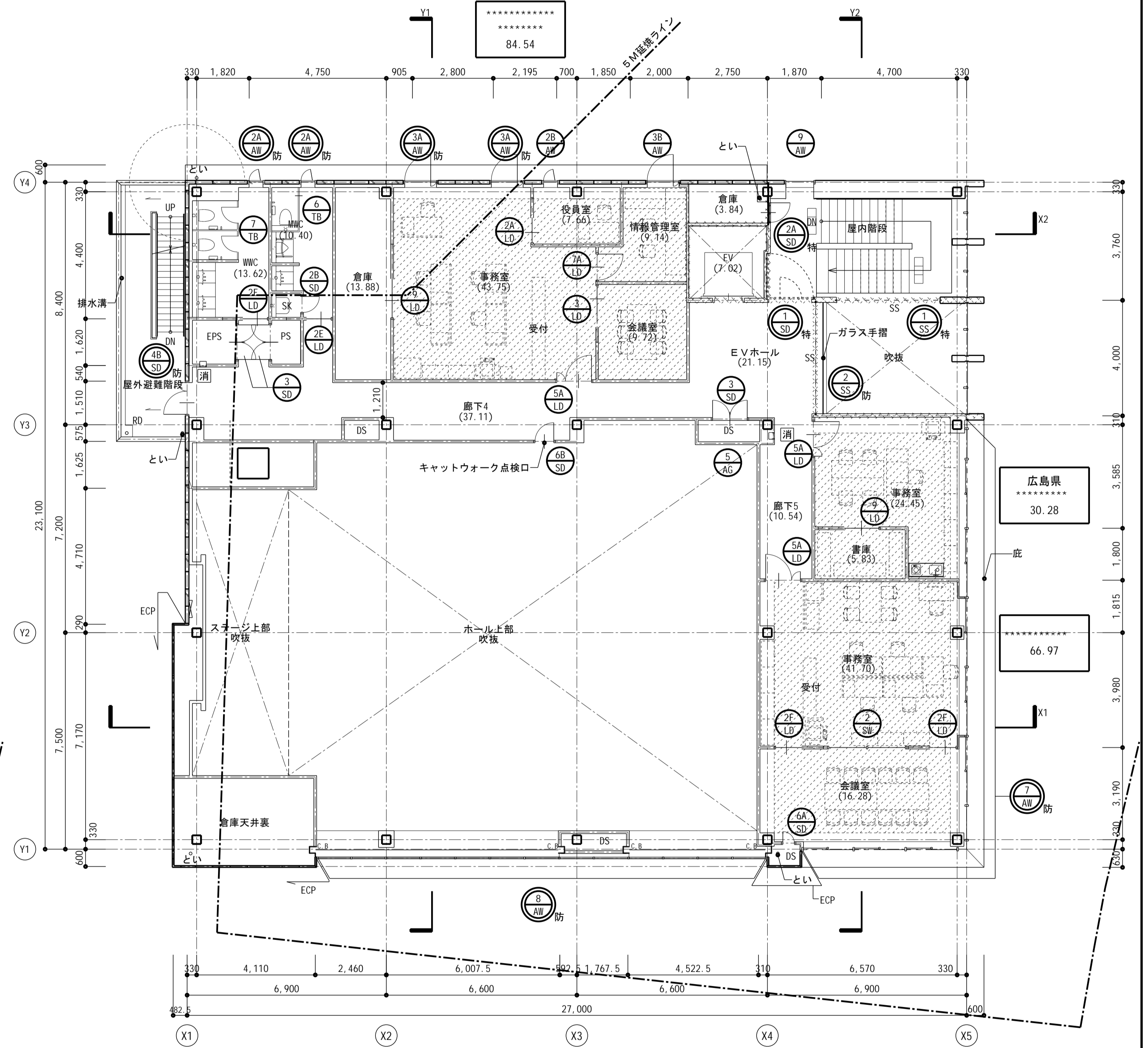
3階平面図
